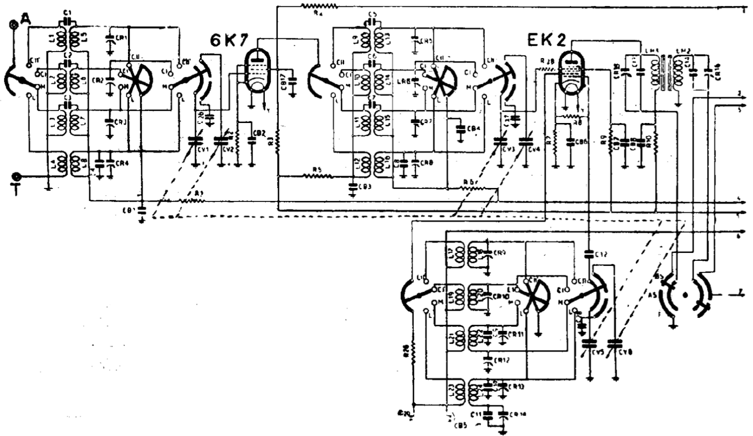
S.A.F.A.R. - MOD. « 542 » PARTI AF - MF
