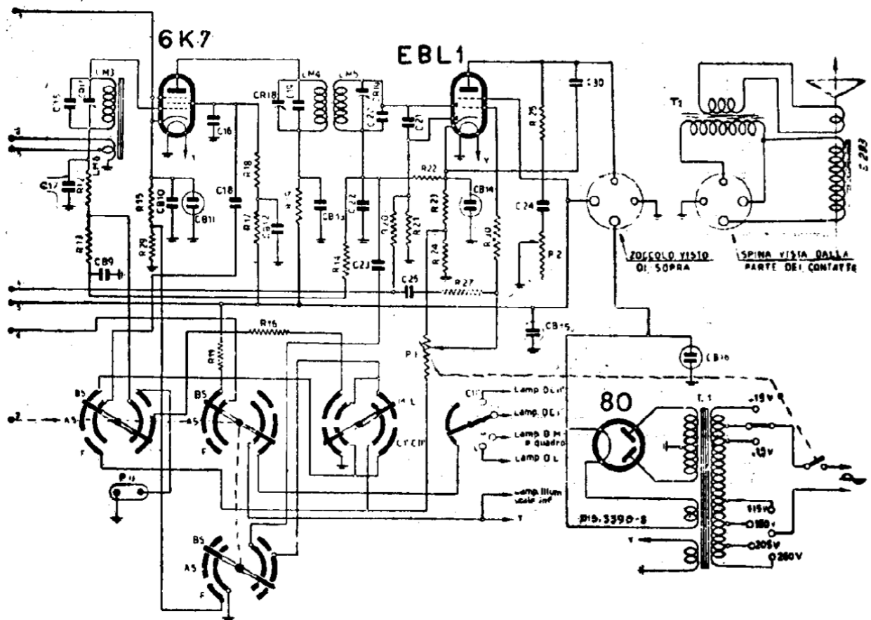
S.A.F.A.R. - MOD. « 542 » - PARTE BF E ALIM.
